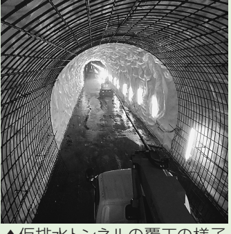
▲仮排水トンネルの覆工の様子
