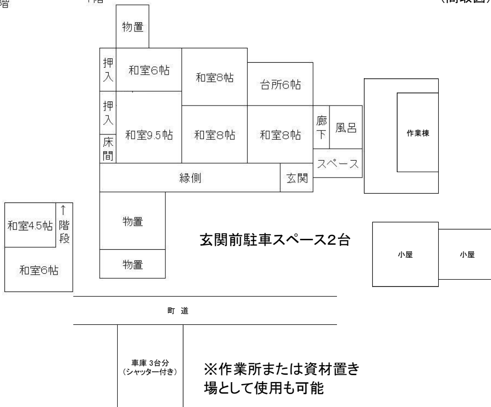
2階 1階 (間取図)
